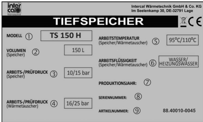
Abb. 2: Muster Typenschild
